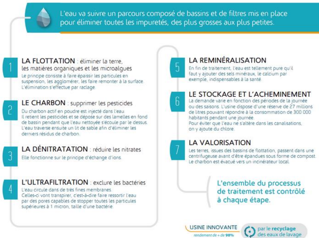
Figure 23 : Les traitements de l'eau brute dans l'usine de Pléven (source : SMAP)
